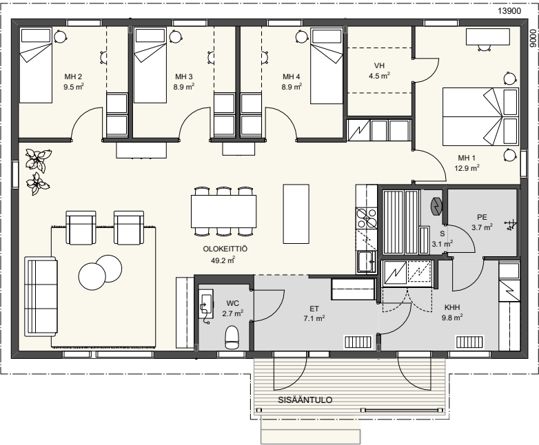
Aisti 125/135 Huoneistoala: 125 m 2 Kerrosala: 135 m 2
