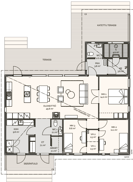
Aisti 122/132 Huoneistoala: 122 m 2 Kerrosala: 132 m 2
